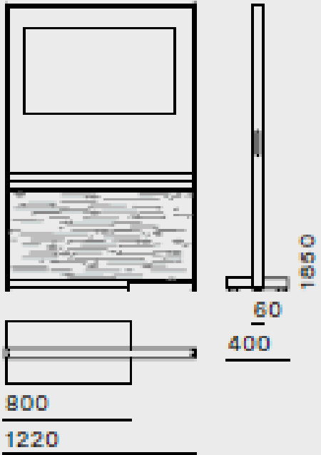
Separatore con scrivania Partition panel with desk
