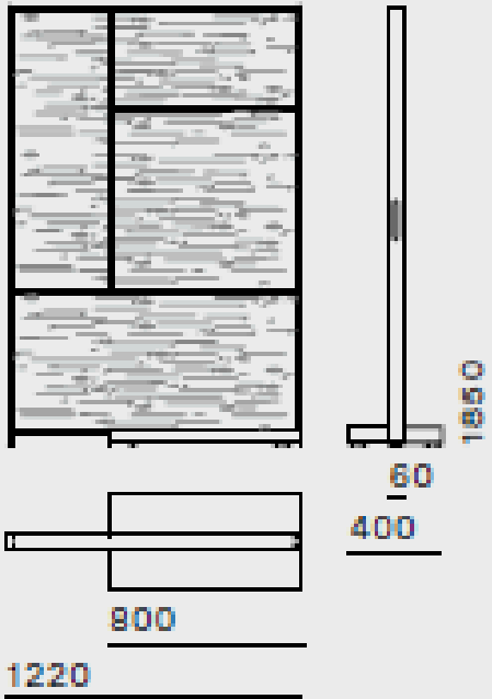
Separatore con ripiani Partition with shelves
